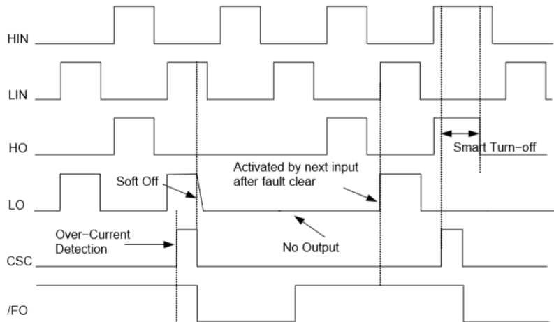
图 9：过流保护时序
