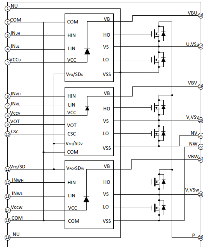
图 1: 模块内部电路示意图
