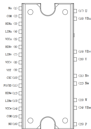
图 2: 模块引脚分布示意图
